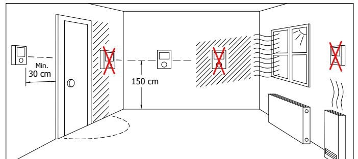
Şekil 42 Oda Termostadının yerleşim konumu
