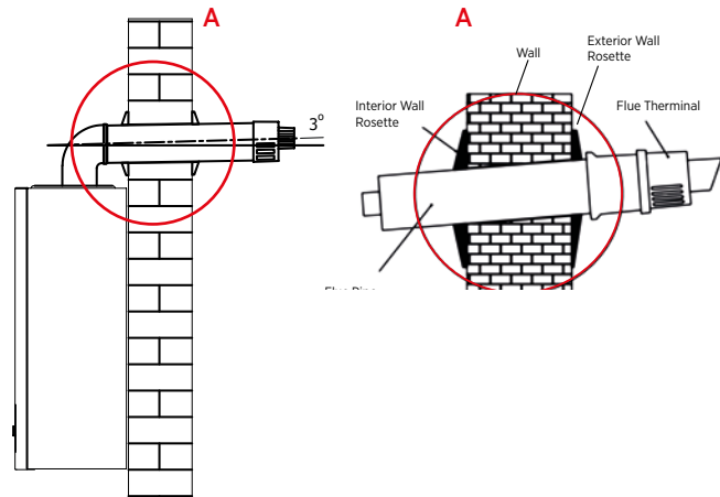
Şekil 27 Yoğuşmalı baca setlerinde, iç baca borusu standart olarak yukarı doğru eğimli olduğundan ayrıca eğim verilmesine gerek yoktur!
