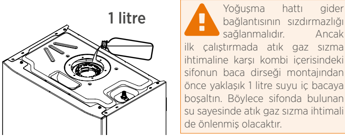
Şekil 15 Yoğuşma sifonunun doldurulması
