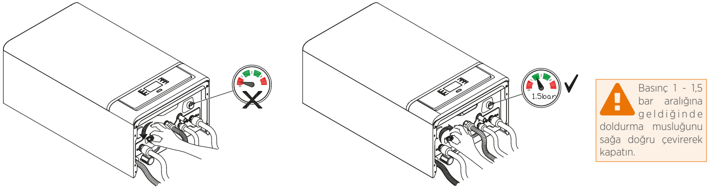
Şekil 10 Kaldifer tesisat suyunun kombinin doldurma vanası ile doldurulması ve basınç kontrolü.
