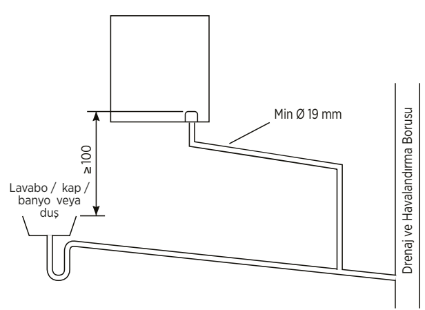
Şekil 17 Alt Seviyede Banyo Drenajına Yoğuşma Suyu Drenaj Borusunun Bağlantısı
