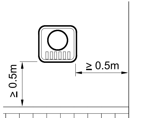
Şekil 39 C Tipi cihazların atık gaz çıkış ağızlarının yana ve alta uzaklığı
