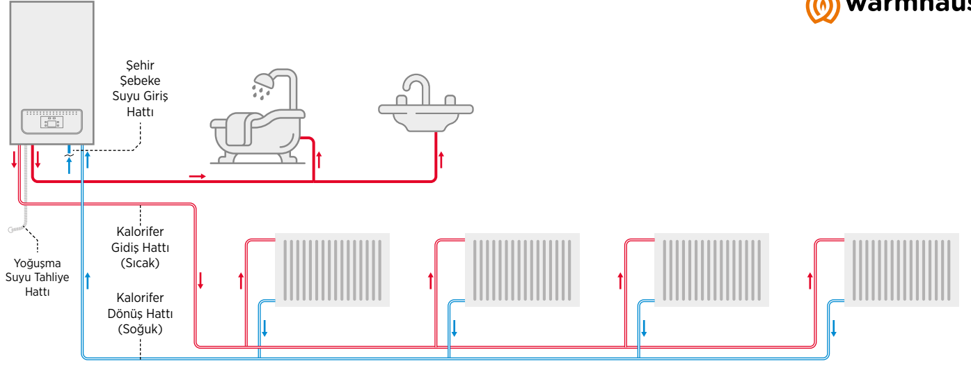
Şekil 12 Çift borulu kombi genel tesisat şeması
