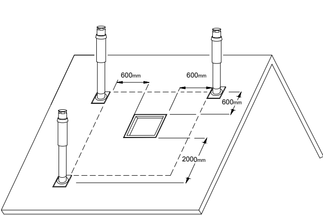
Şekil 38 Atık gaz bacasının açılabilir çatı penceresine olan konumları ve mesafeleri
