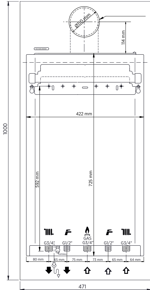
Şekil 1 Montaj şablonu
