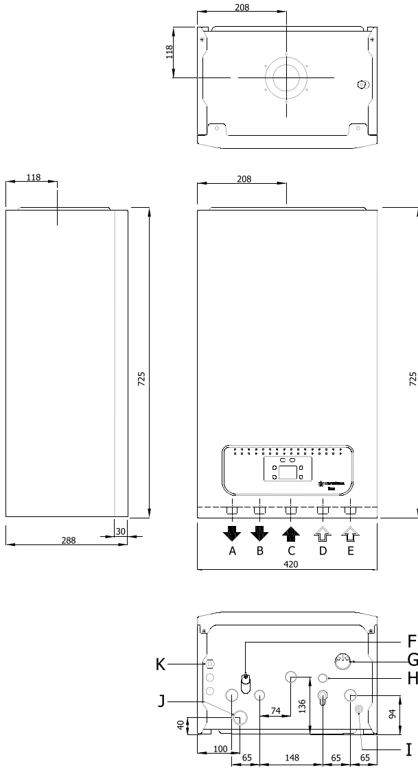
Şekil 7 Ewa Kombi boyutları ve bağlantıları
