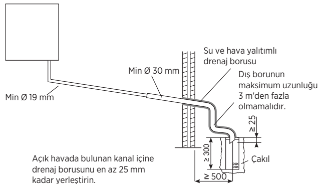
Şekil 18 Yoğuşma Suyu Drenaj Borusunun Dış Bağlantısı
