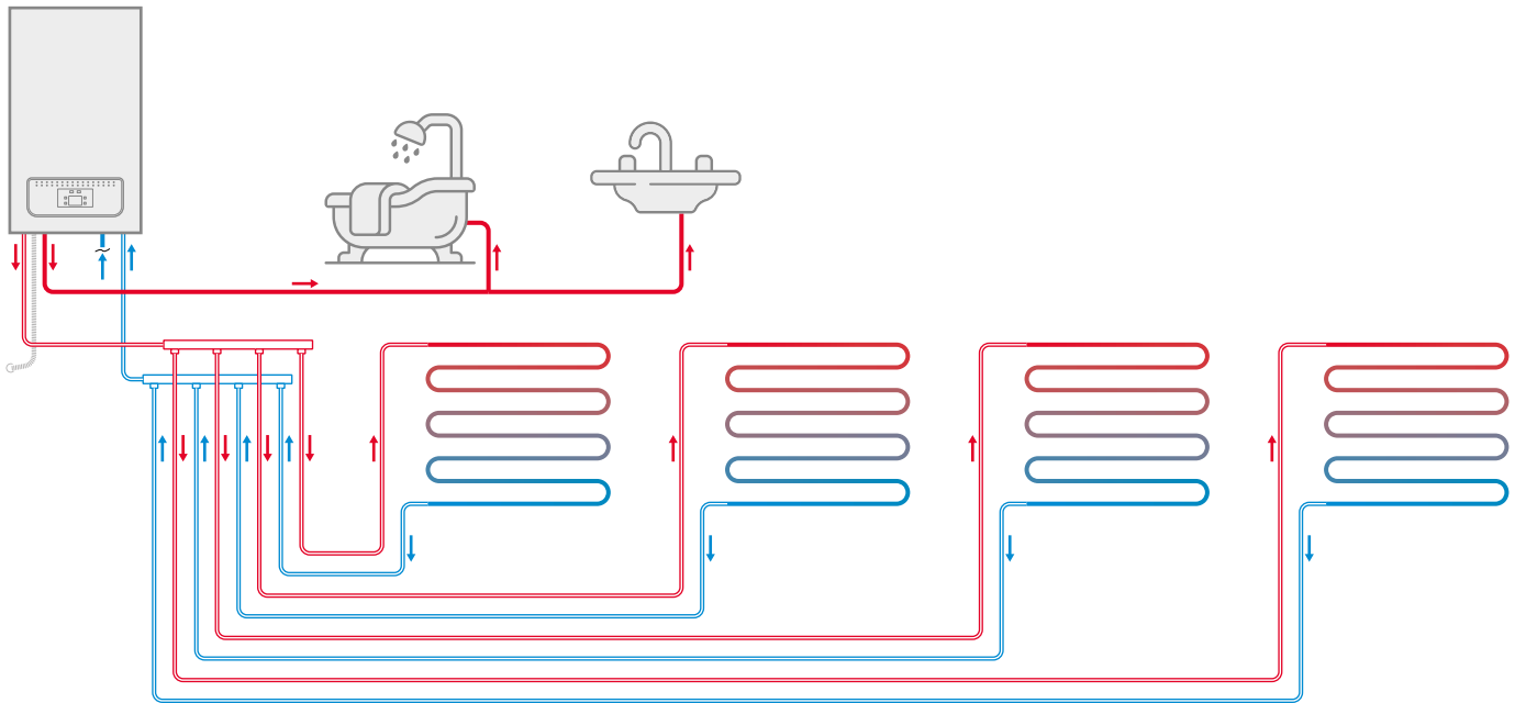
Şekil 14 Mobil boru dağıtım sistemli kombi yerden ısıtma genel tesisat şeması
