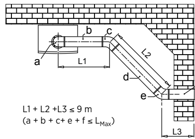
Şekil 30 III. Tek 90° ve iki 45° dirsekli örnek yoğuşmalı kombi baca tesisatı
