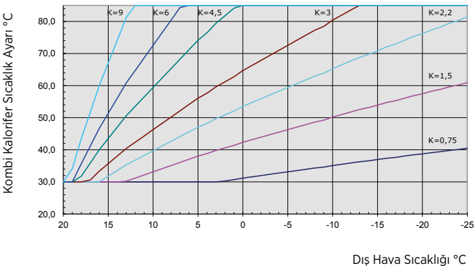
Şekil 45 Dış hava sıcaklık sensörü çalışma eğrileri
