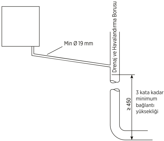
Şekil 16 Yoğuşma Suyu Drenaj Borusunun Dahili Drenaj ve Havalandırma Borusuna Bağlanması
