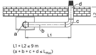
Şekil 29 II. İki 90° dirsekli örnek baca tesisatı
