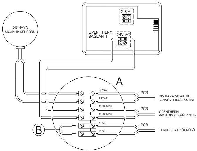
Şekil 41 Kombi oda termostadı ve dış hava sıcaklık sensörünü bağlantıları
