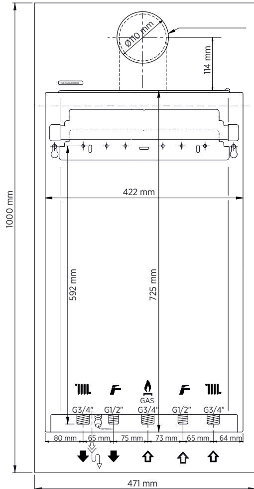
Şekil 1 Montaj şablonu
