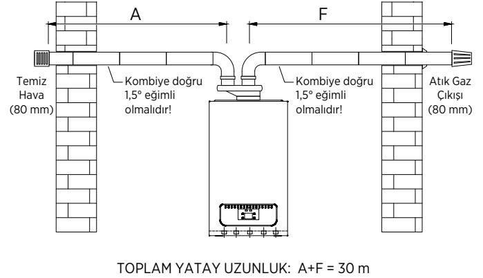
Şekil 34 Ayrık baca tipi (hermetik) Yatay Montaj Mesafeleri
