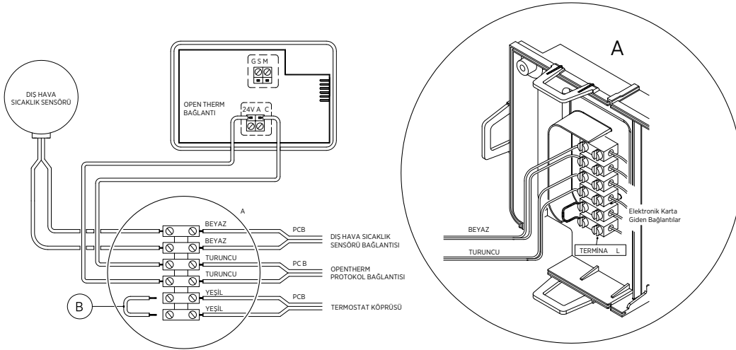
Şekil 41 Kombi oda termostadı ve dış hava sıcaklık sensörünü bağlantıları
