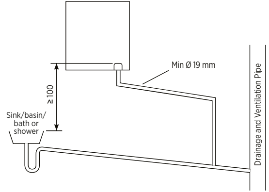
Şekil 17 Alt Seviyede Banyo Drenajına Yoğuşma Suyu Drenaj Borusunun Bağlantısı
