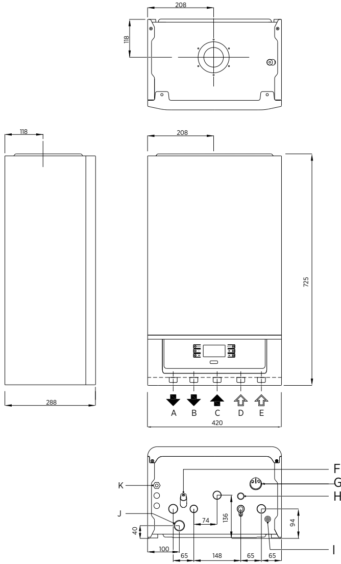
Şekil 7 EnerwaPlus Kombi boyutları ve bağlantıları
