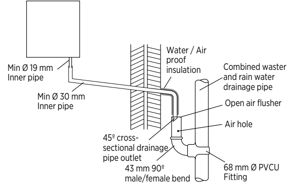
Şekil 21 Yoğuşma Drenajının Drenaj ve Havalandırma Borusuna Bağlanması
