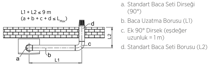
Şekil 29 II. İki 90° dirsekli örnek baca tesisatı
