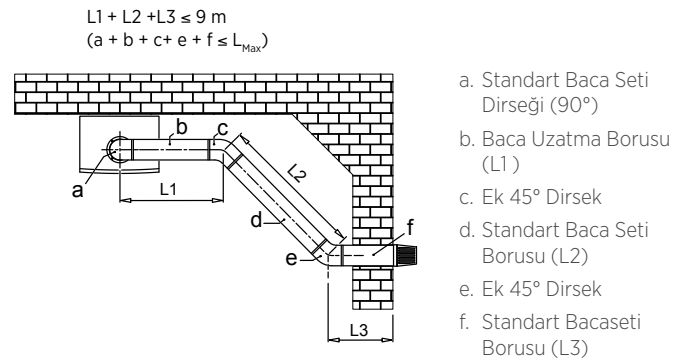
Şekil 30 III. Tek 90° ve iki 45° dirsekli örnek yoğuşmalı kombi baca tesisatı
