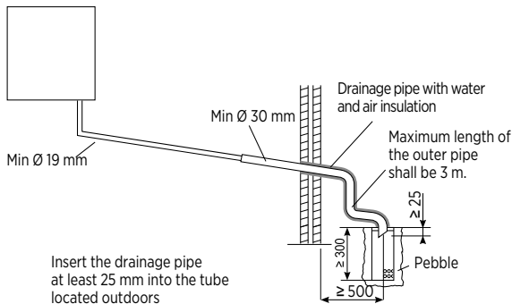
Şekil 18 Yoğuşma Suyu Drenaj Borusunun Dış Bağlantısı
