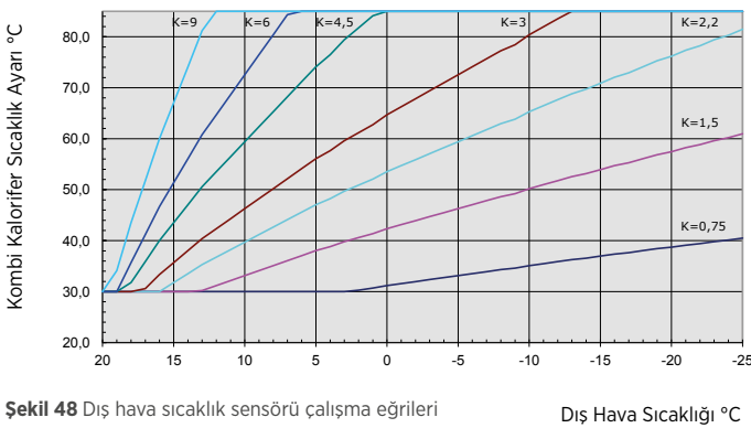
Şekil 48 Dış hava sıcaklık sensörü çalışma eğrileri
