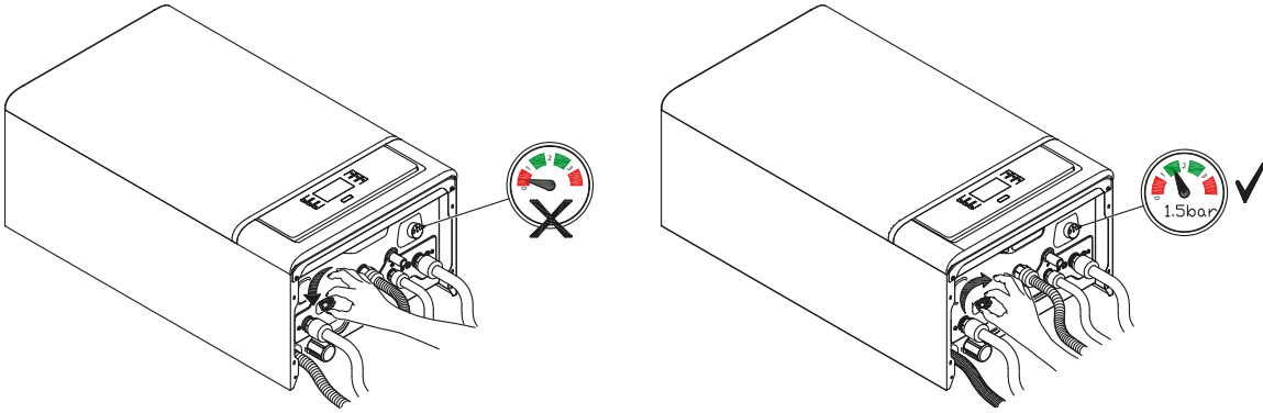
Şekil 10 Kaldırma tesisi suyunun kombin doldurma vanası ile doldurulması ve basınç kontrolü.
