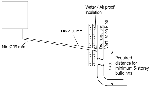
Şekil 20 Yoğuşma Drenajının Drenaj ve Havalandırma Borusuna Bağlanması
