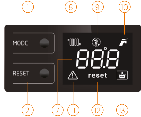
Şekil 44 Enerwa kombilerin kumanda paneli ekranı
