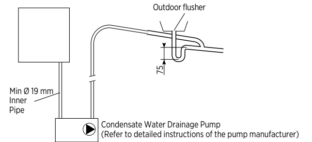
Şekil 19 Yoğuşma Suyu Drenaj Borusunun Tipik Bağlantı Yöntemi (Pompa üreticisinin ayrıntılı talimatlarına bakın)
