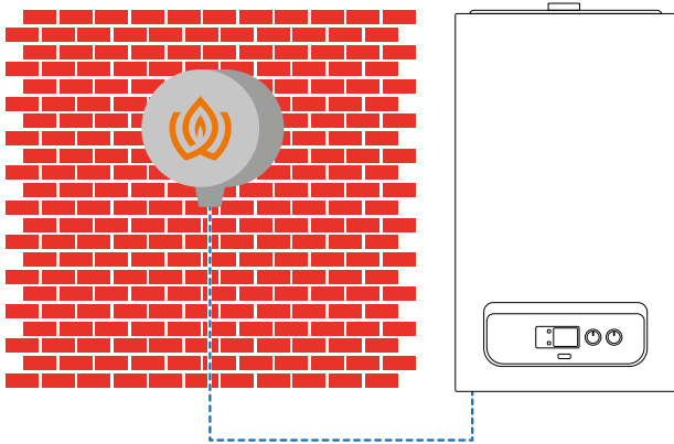
Şekil 47 Dış hava sıcaklık sensörü ve kombi bağlantısı
