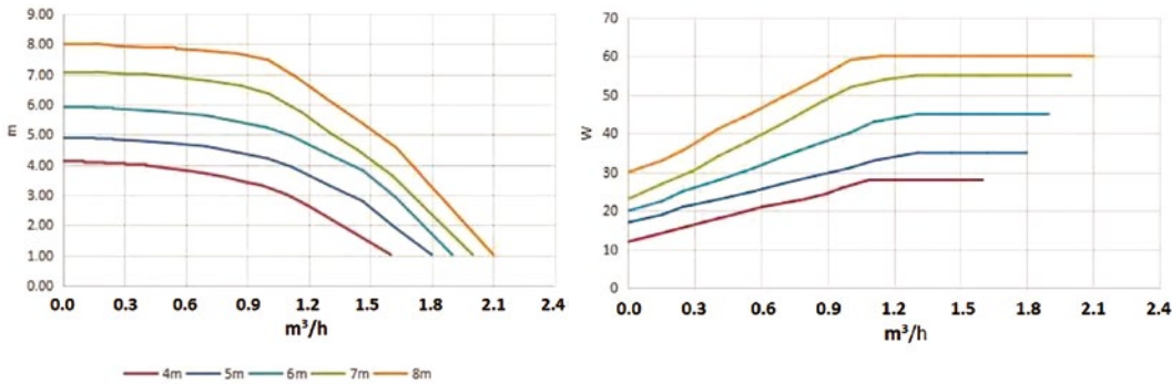
Şekil 11 Enerwa kombiler için kullanılan Otomatik Güç Ayarlı ve Otomatik Hava Purjör Pompa Debi/Basınç ve Güç Tüketim Grafikleri
