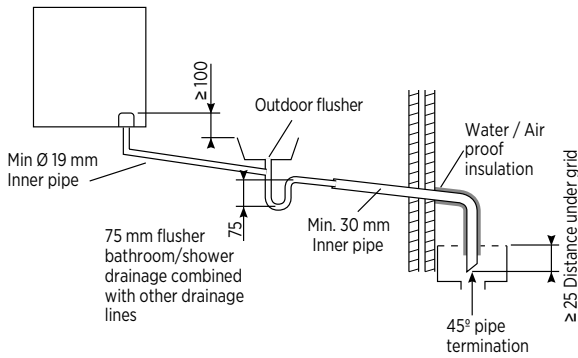
Şekil 22 Yoğuşma Drenajının Lavabo, Küvet veya Duş Drenaj Borusu ile Yağmur Drenaj Hattına Bağlanması
