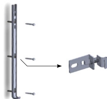
Radyatör tapası
