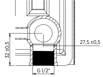
Detay B
