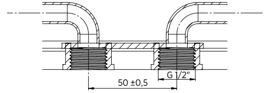
Detay A
