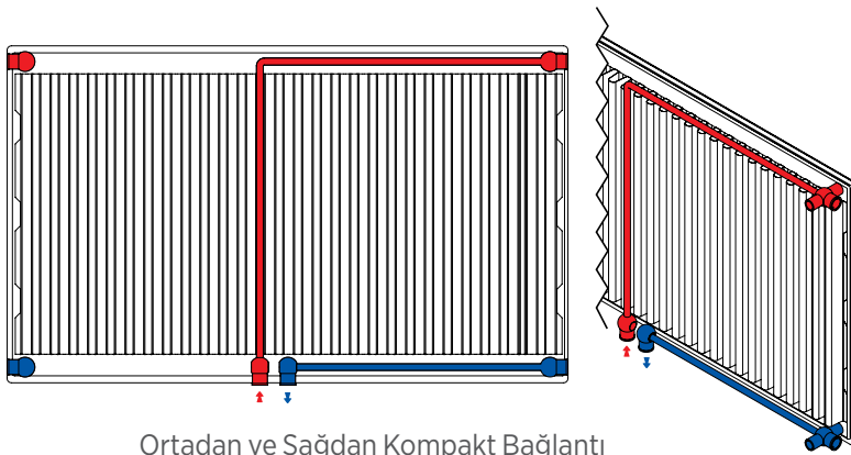
Ortadan ve Sağdan Kompakt Bağlantı
