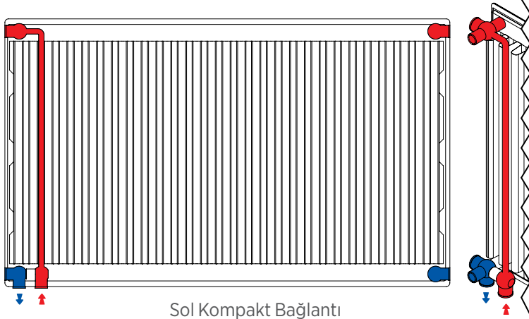
Sol Kompakt Bağlantı
